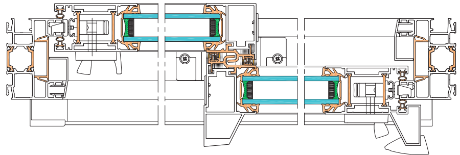
Coupe horizontale
