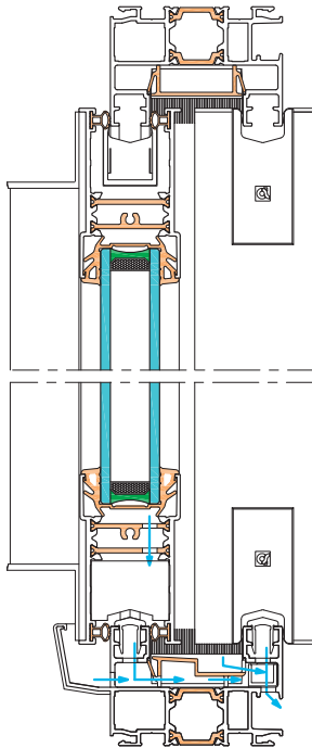
Coupe verticale
