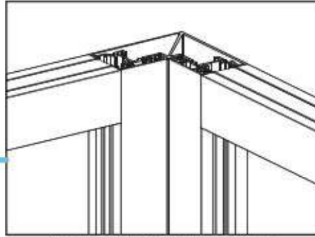
Assemblage cadre et poteau 2 départs
